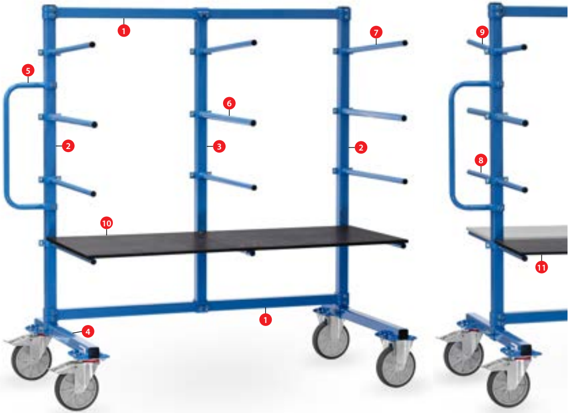
Eléments pour chariots à barres de portée horizontales
